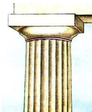
kapitel dorycki
